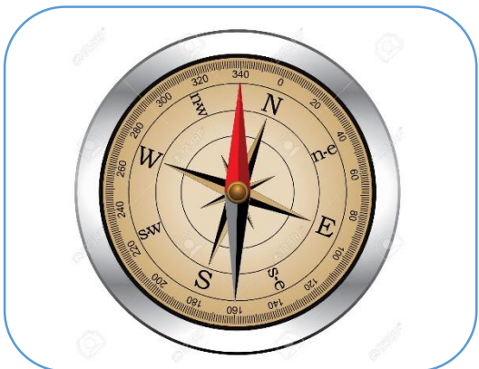
КОМПАС
